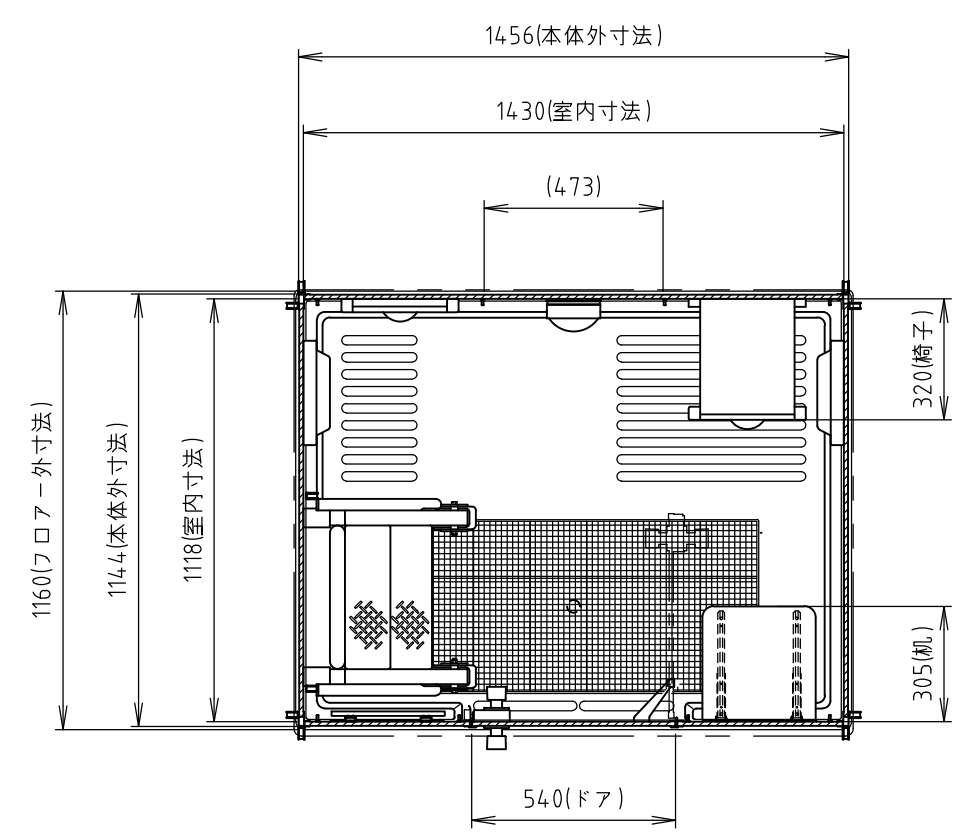
平面図 (内装)
